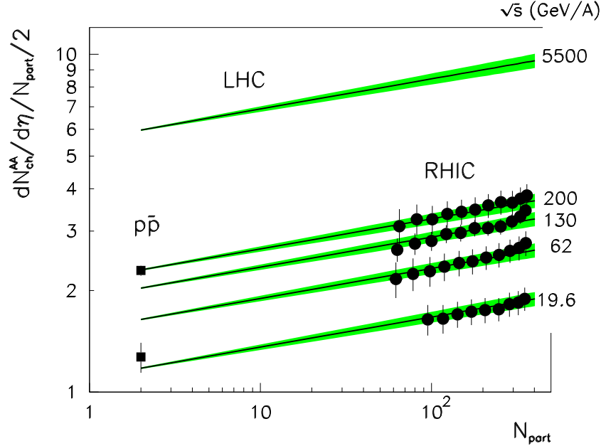
Рис. 3: Зависимость множественности частиц от центральности столкновений и от энергии величины dN^{ch}/d\eta(0) , нормированной на число пар участвующих нуклонов N_{\text{part}}/2 (данные PNOBOS [1]). Затененные области — предсказания модели насыщения [18].
