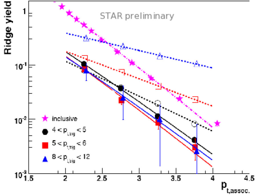
Рис. 31: Выход частиц в области шлейфа (заполненные значки) и в области пика от адронной струи (полые значки) в зависимости от p_{T}^{\text{assoc}} при различных значениях p_T^{\text{trig}} для центральных 0 \div 5\% AuAu-столкновений [120]. Инклюзивный спектр обозначен звездочками.
