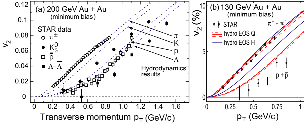
Рис. 9: Параметр эллиптического потока v_2 (а) для \pi^+ -, \pi^- -, K_s^0 -мезонов, антипротонов, \Lambda -гиперонов при 200 ГэВ в AuAu-столкновениях [40] (пунктирные кривые — гидродинамическая модель), Параметр эллиптического потока v_2 (б) при 130 ГэВ и расчеты гидродинамической модели для фазового перехода адроны-кварки (EOSQ) и для адронного газа (EOSH).
