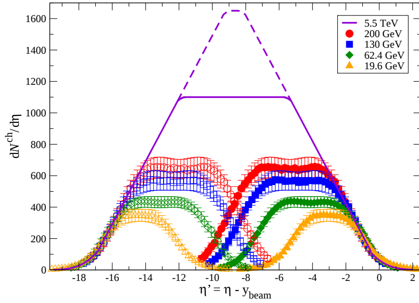
Рис. 2: Множественность заряженных частиц как функция псевдобыстроты \eta' = \eta - y_{\text{beam}} в AuAu-столкновениях при различных энергиях в системе центра масс от \sqrt{s} = 19.6 ГэВ до \sqrt{s} = 5.5 ТэВ. Данные приведены в системе покоя одного из сталкивающихся ядер с зеркальным отражением для другого ядра [21, 22]. Экстраполяция для ЛНС приведена в двух вариантах: 1) продолжение предельной фрагментации и 2) трапециидальная форма.
