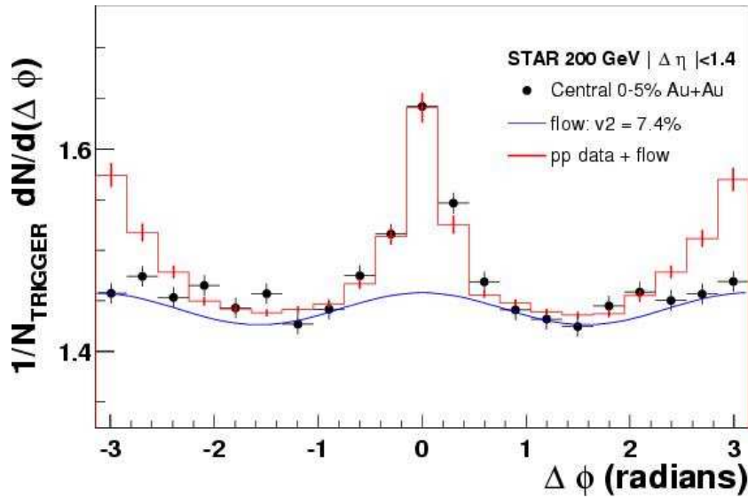
Рис. 23: Двухадронные азимутальные корреляции для pp -столкновений (гистограмма) и для центральных AuAu -столкновений (точки) при \sqrt{s} = 200 А ГэВ. Плавная кривая — фон.
