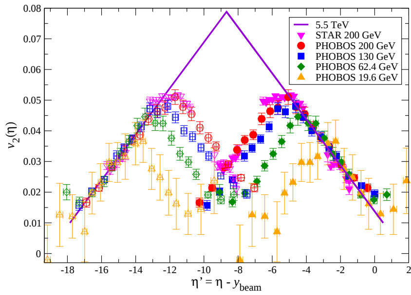
Рис. 7: Зависимость эллиптического потока v_2 от \eta' = \eta - y_{\text{beam}} для центральных 0 ÷ 40%.
