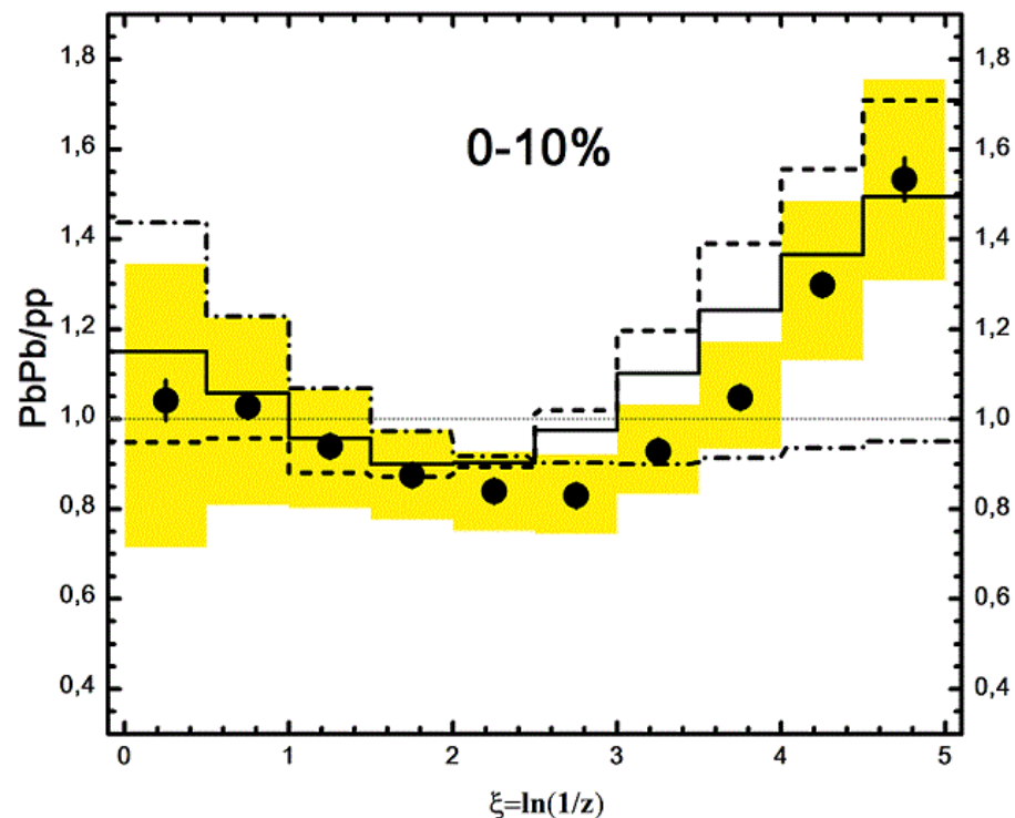
Функция фрагментации:
