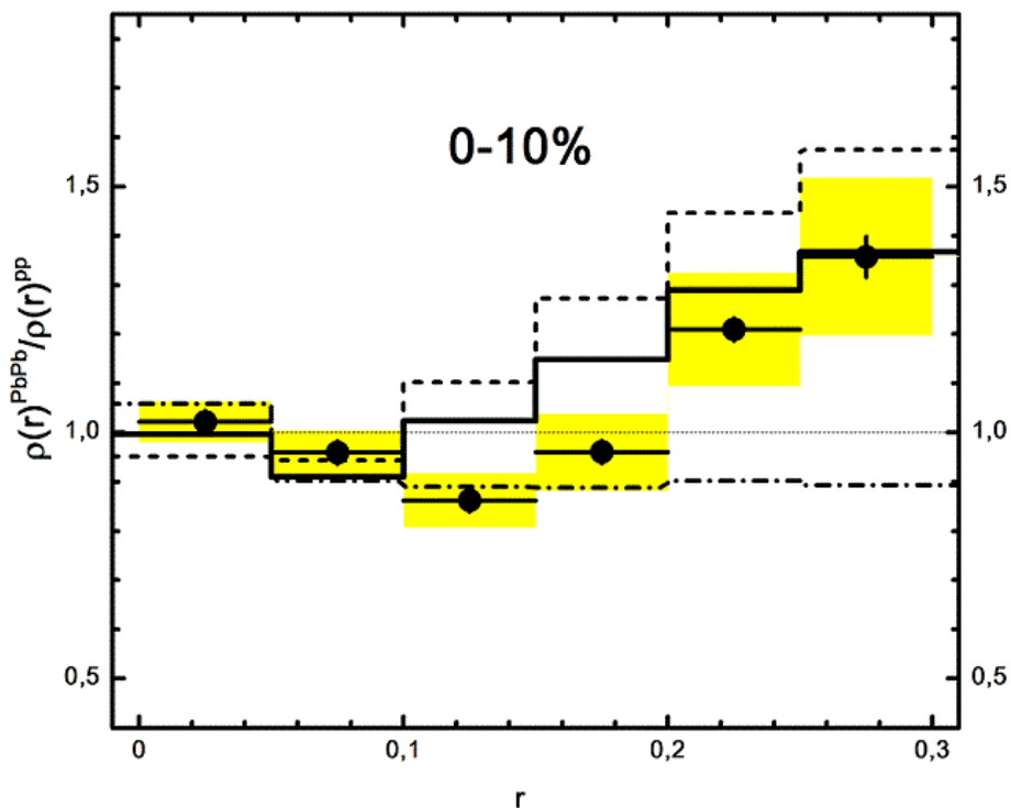
Форма струй:
